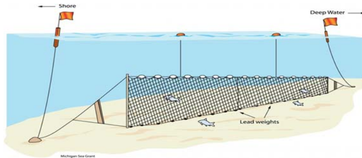
Fig. 32 : Gill net
