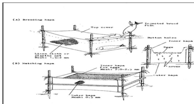
Fig.8: Hapa
